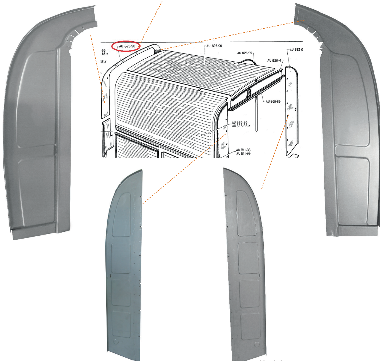
52011342 TOLE DE FERMETURE ARRIERE GAUCHE AK250 / AZU
